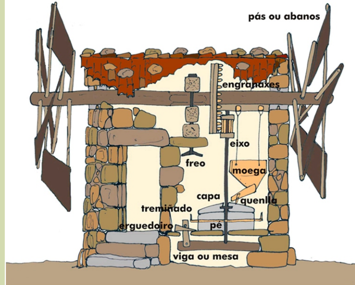
Esquema dun muíño de vento de Catoira
